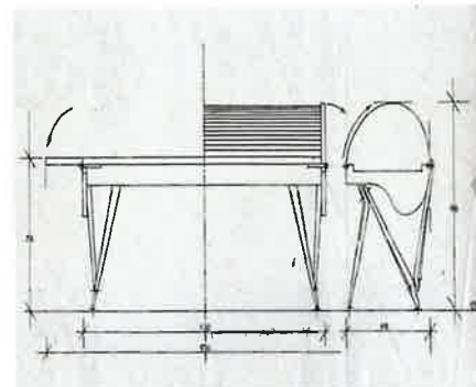
10. Scrivania a cilindro con chiusura a serrandina scorrevole, fianchi a ribalta e sostegno a traliccio scolpito in legno laccato nero, ideata per Casa Mollino, 1946/1947
