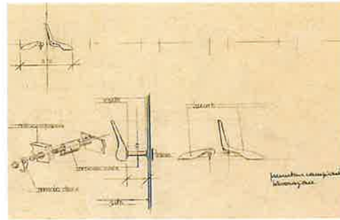
7. Appendiabiti in legno scolpito laccato nero. Gancio, distanziali e dadi di fissaggio a parete in ottone lucido, ideato per Casa Minola, 1944/1946
