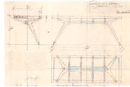
5. Tavolo in rovere scolpito in giunti in ottone e piano di cristallo temprato in tre pezzi poggiati su profili interni in acciaio, ideata per Casa Albonico, 1944
