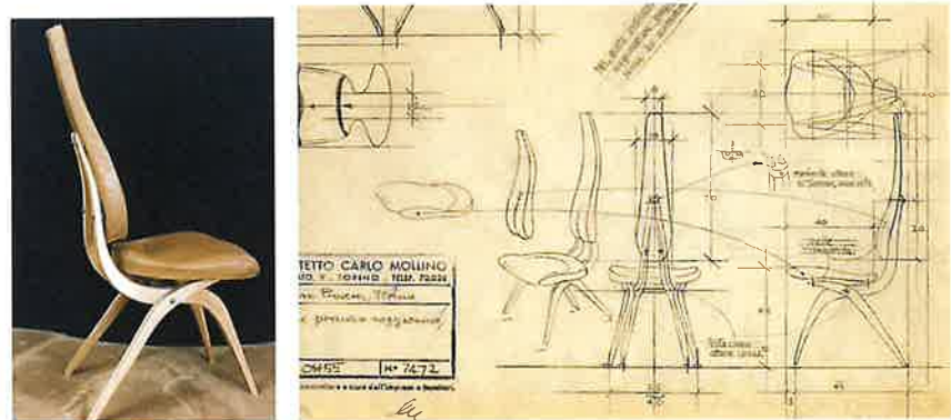
27. Sedia in acero naturale scolpito rivestito in pelle. Le gambe anteriori si prolungano formando il supporto, ideata per la sala da pranzo di Casa Provera (Torino), 1956
