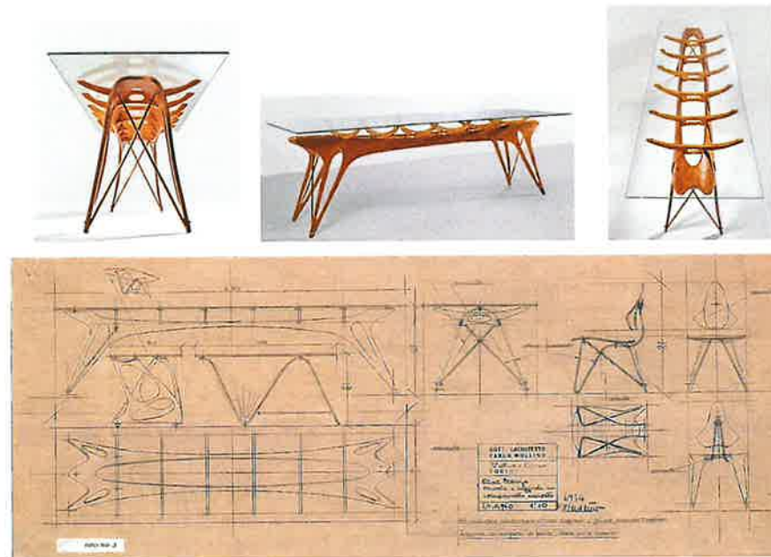
18. Tavolo con struttura in compensato di acero naturale curvato e lucidato, giunti di ottone spazzolato e piano in cristallo temperato, ideato per la mostra "Italy at work" a New York, 1950
