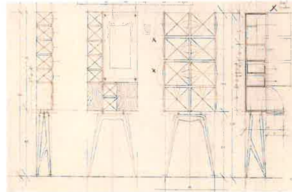
6. Credenza in legno bugnato con struttura di supporto a traliccio in legno scolpito lucidato e raccordi in bronzo sagomato, ideata per Casa Albonico, 1944
